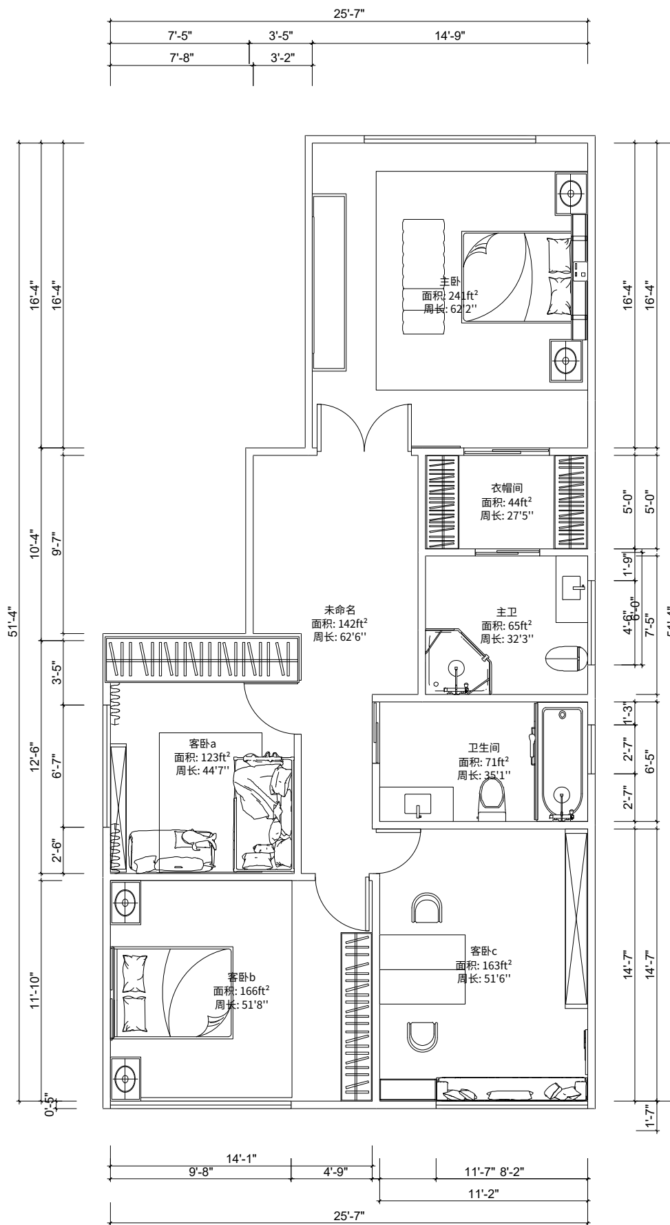
平面布置(1:85)
