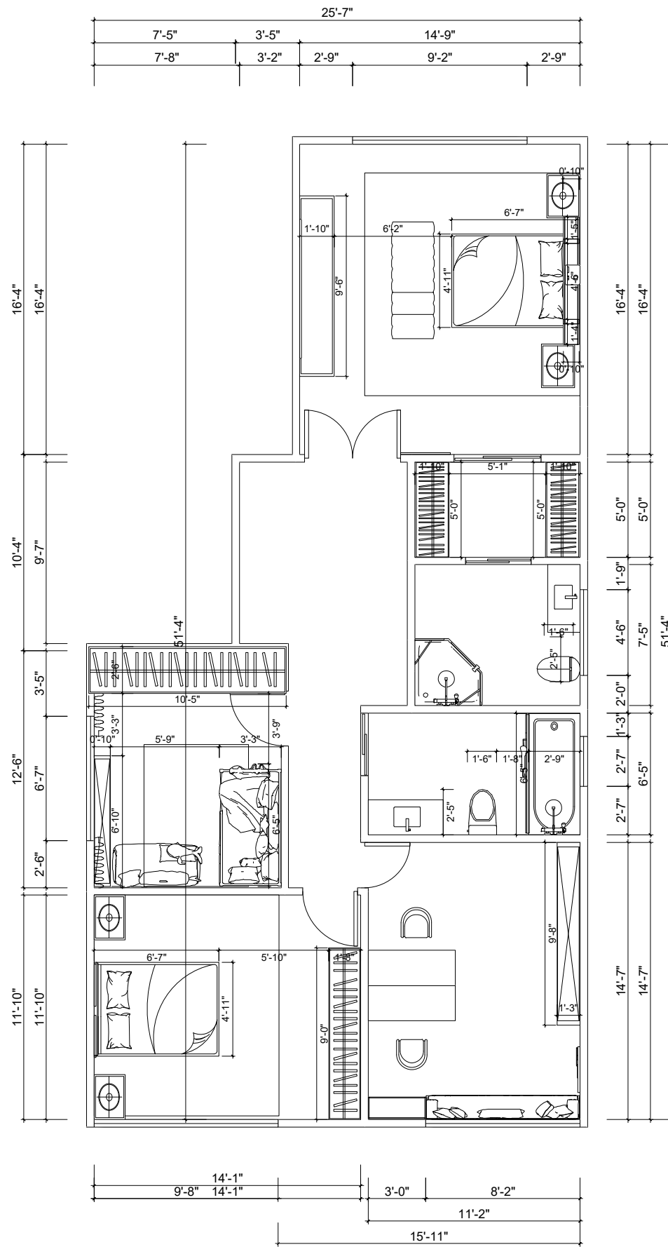
家具尺寸(1:85)
